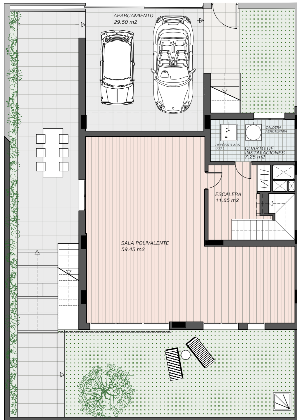
PLANTA SÓTANO
