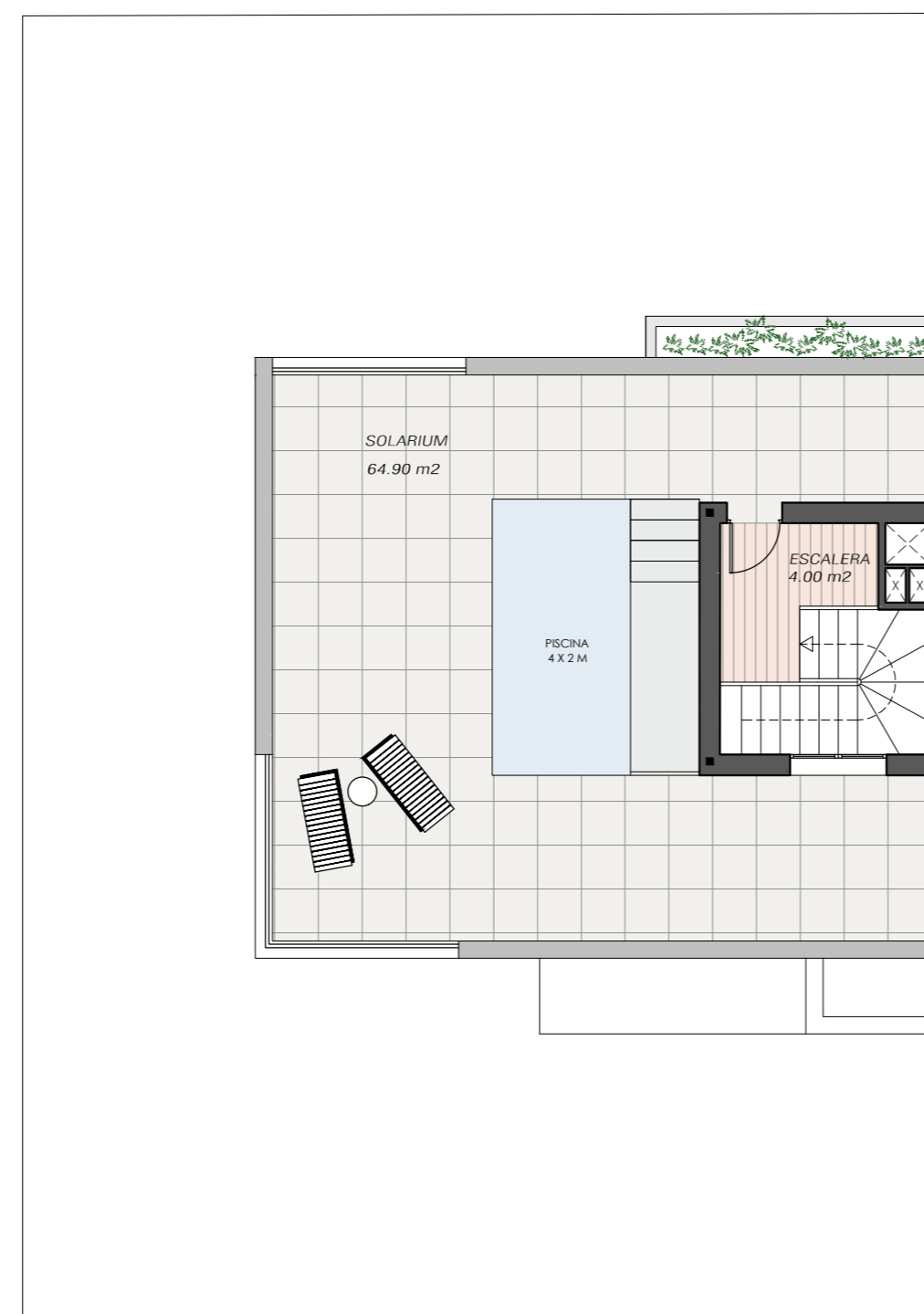
PLANTA CUBIERTA
