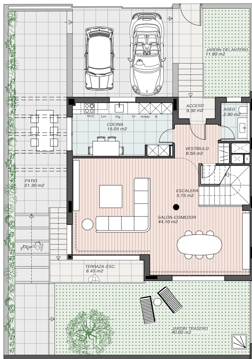
PLANTA BAJA
